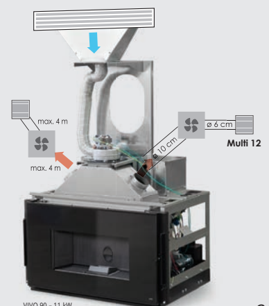
VIVO 90 - 11 kW
