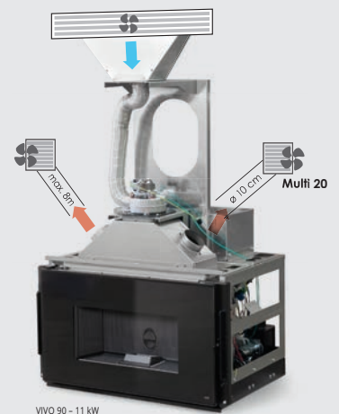
VIVO 90 - 11 kW
