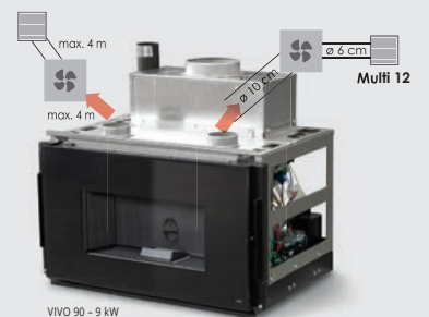
VIVO 90 - 9 kW
